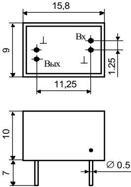
Рис.2 Корпус пластмассовый
