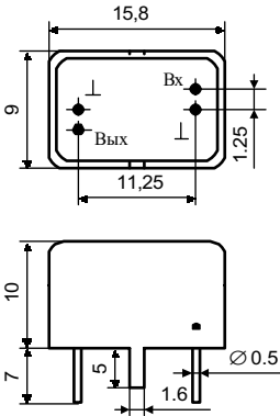
Рис.1 Корпус металлический
