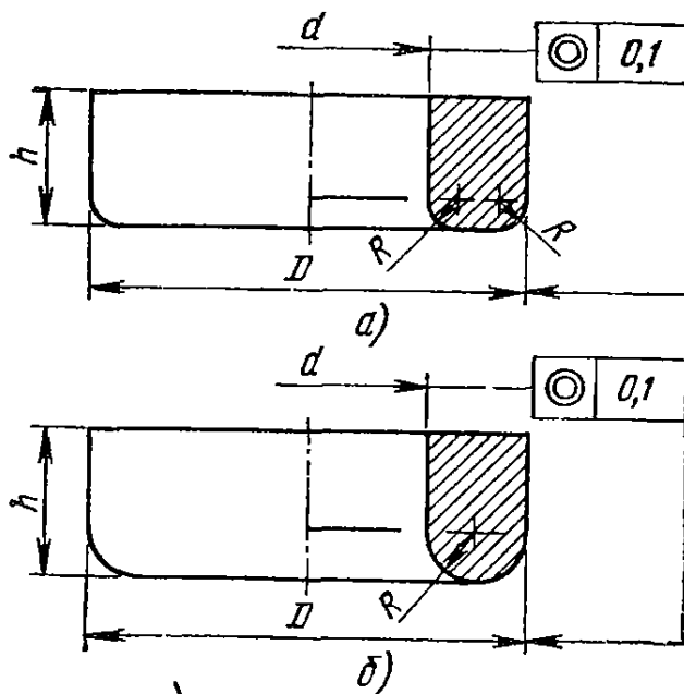
Рис. 6.35. Сердечники кольцевые:
