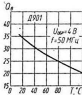
Зависимость добротности от температуры
