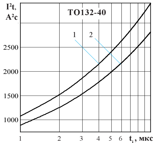
Рисунок 9 - Зависимость защитного показателя I^2t от длительности импульса тока t_1 при исходной температуре структуры T_j = 25\text{ }^\circ\text{C} (1) и максимальной температуре T_{jm} (2)
