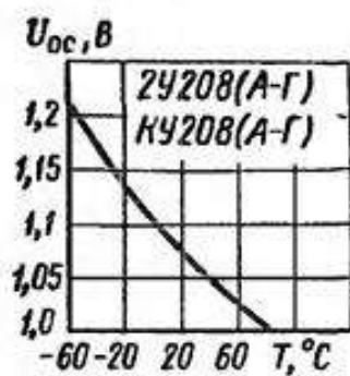
Зависимость напряжения в открытом состоянии от температуры
