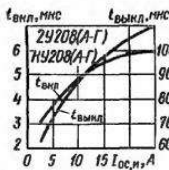
Зависимости времени включения и выключения от импульсного тока
