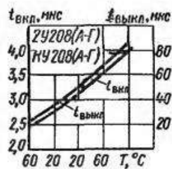
Зависимости времени включения и выключения от температуры
