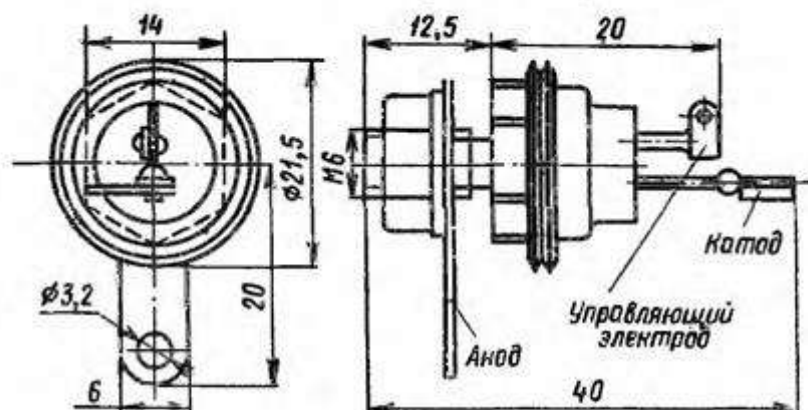
2У208(А-Г), КУ208(А-Г)
