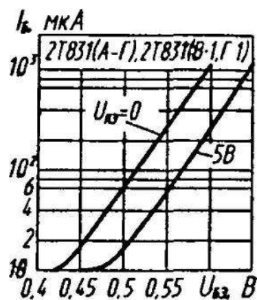
Входные характеристики
