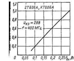
Зависимость относительной выходной мощности от входной.
