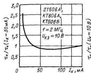
Зависимость относительной постоянной времени цепи обратной связи от тока коллектора
