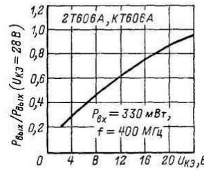
Зависимость относительной выходной мощности от напряжения коллектор-эмиттер.
