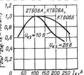
Зависимость модуля относительного коэффициента передачи тока от тока коллектора
