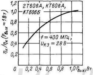
Зависимость относительного коэффициента полезного действия от выходной мощности
