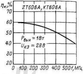
Зависимость коэффициента полезного действия от частоты
