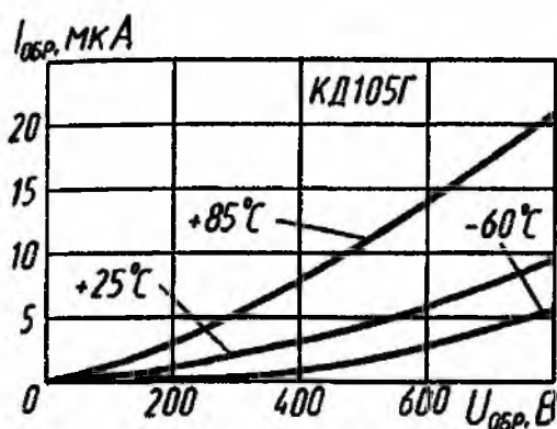
Зависимости обратного тока от напряжения
