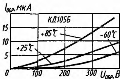
Зависимости обратного тока от напряжения
