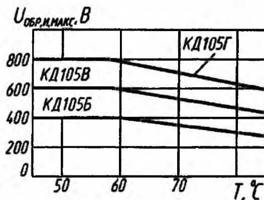
Зависимости допустимого обратного напряжения от температуры
