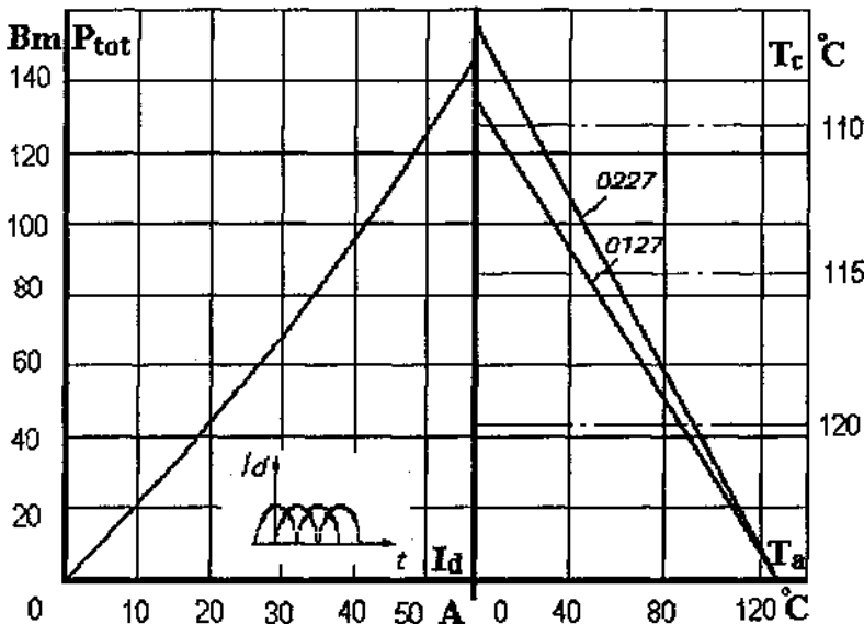
Рис. 2. 23.* Зависимость допустимой суммарной рассеиваемой мощности и допустимого выпрямленного тока трех модулей МТТ4/3 - 40 на охладителях О127 и О227 от температуры окружающей среды и температуры корпуса при естественном охлаждении
