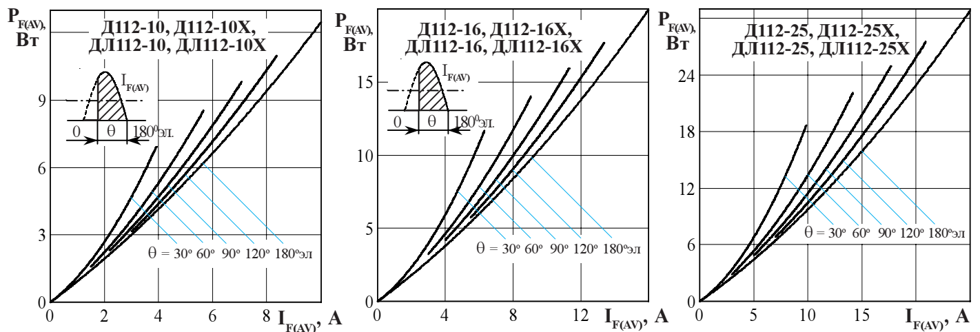
Рисунок 6 - Зависимость средней прямой рассеиваемой мощности P_{F(AV)} от среднего прямого тока I_{F(AV)} синусоидальной формы частоты f = 50 Гц
