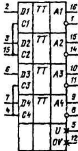
Условное графическое обозначение К133ТМ7
