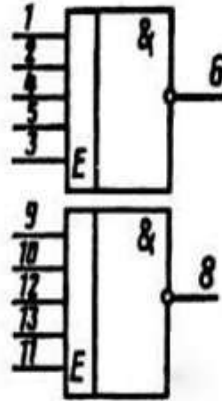
Условное графическое обозначение К511ЛА4
