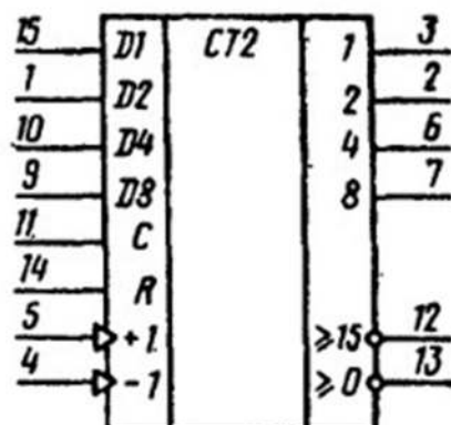
Условное графическое изображение K155IE7, KM155IE7
