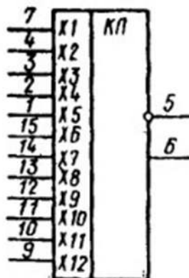
Условное графическое обозначение К155КП7, КМ155КП7, КБ155КП7-4
