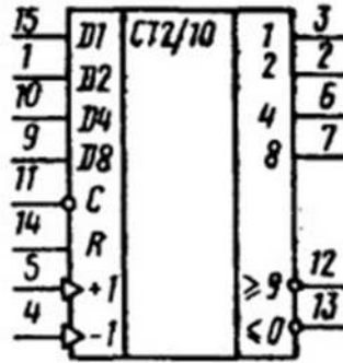
Условное графическое изображение К155ИЕ6, КМ155ИЕ6
