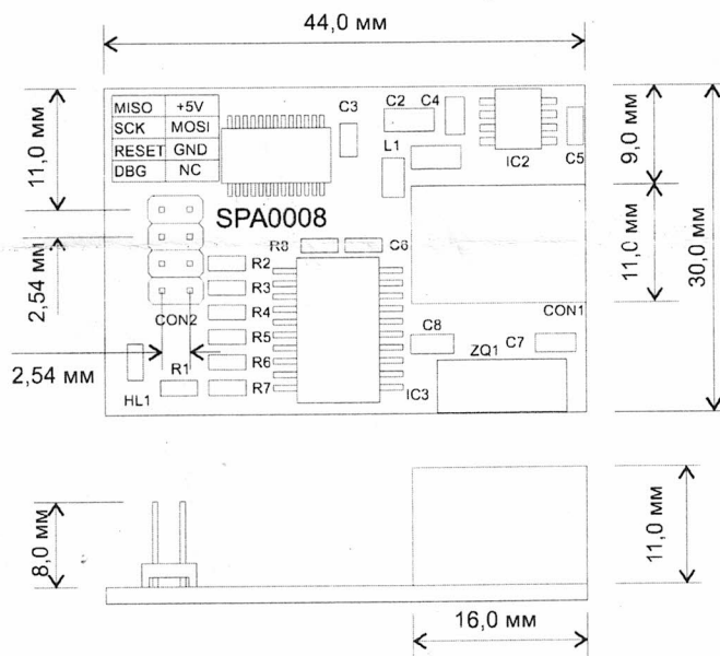
Габаритный чертёж
