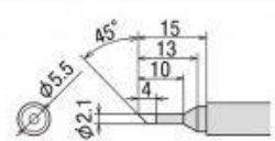
PX-2RT-2CR
