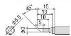
PX-2RT-3CR
