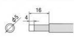
PX-2RT-5CR
