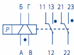
Схема электрическая принципиальная РПС 45, РПС 45-1
