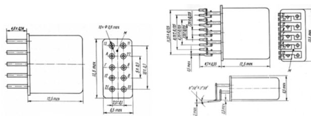
Габаритные размеры РПС 45 РПС 45-1
