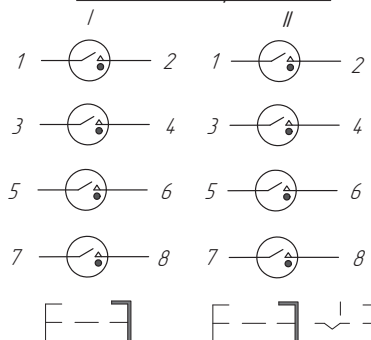
Схема электрическая
