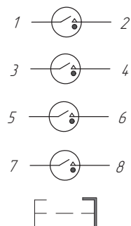
Схема электрическая
