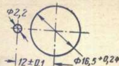
Рис. 26. Общий вид, габаритные и установочные размеры выключателей ВБТ-1, ВБТ-2, ВБТ-4 и рычажных переключателей ТВ1-1, ТВ1-2, ТВ1-3
