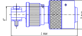
Вилка (розетка) кабельная с прямым кожухом
